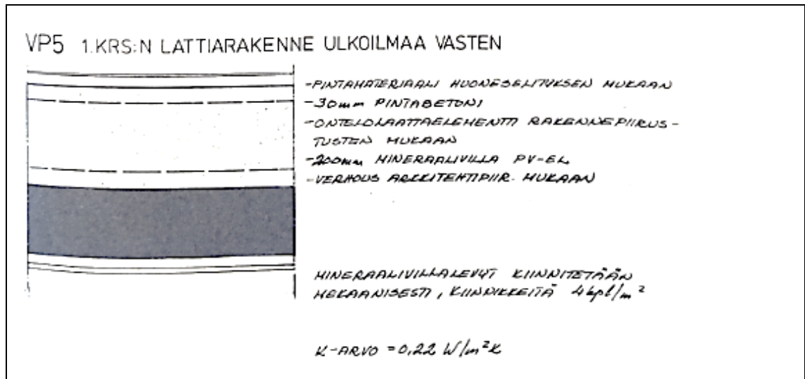
Kuva 5.49. Ulkoilmaa vasten oleva lattiarakenne.
