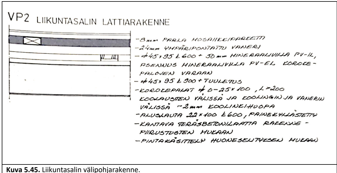
Kuva 5.45. Liikuntasalin välipohjarakenne.
