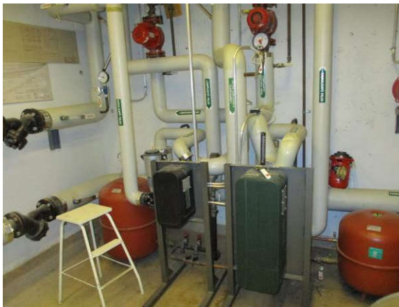
Lämmönjakokeskuksen v. 1995 osa
