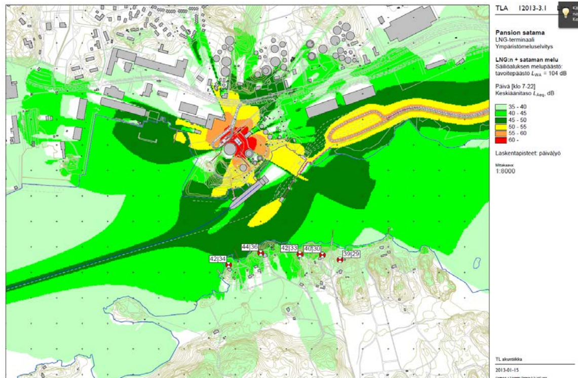
KUVA: LNG:n ja sataman melu, säiliöaluksen melupäästö: tavoitepäästö L_{WA} = 104 dB, TL akustiikka
