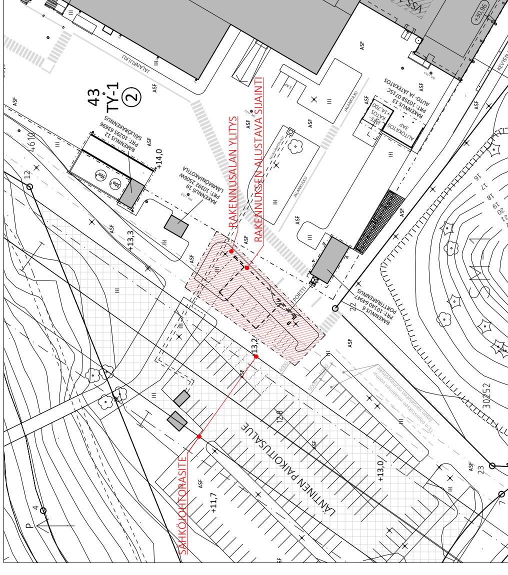
ASEMPIIRROSOTE, 1:500
