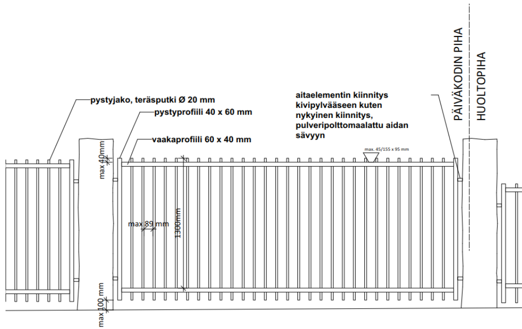
Ote projektiosta A, 1:20 Uudet aitaelementit, rakennevahvuudet ja -profiilit kuten nyk.
