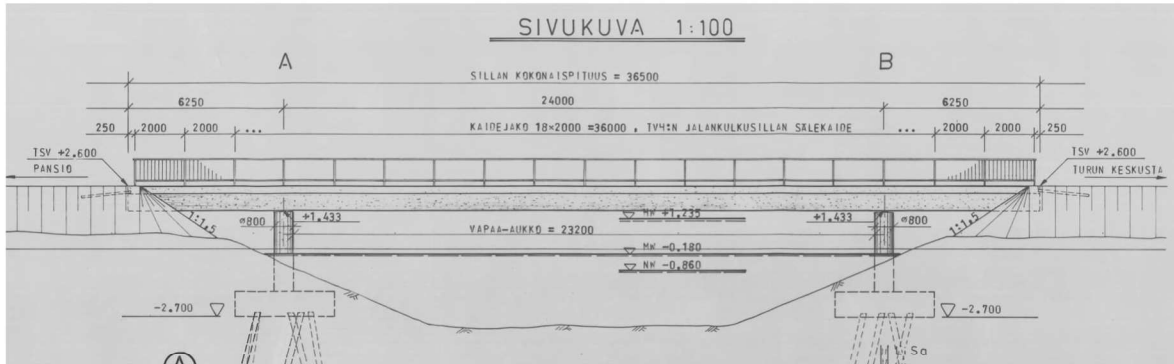
Kuva 2: Sillan yleispiirustus, pituusleikkaus (v.1979)
