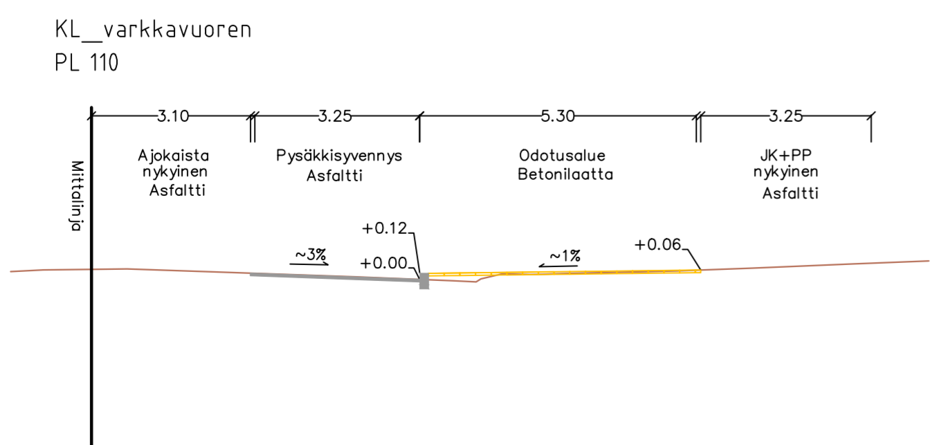
Tyypipoikkileikkaus 1:100 Linja-autopysäkki 33 Markulantie
