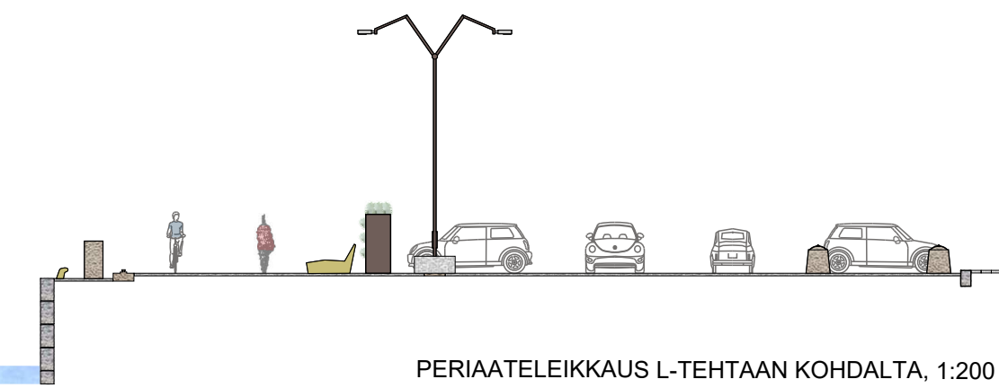
PERIAATELEIKKAUS L-TEHTAAN KOHDALTA, 1:200
