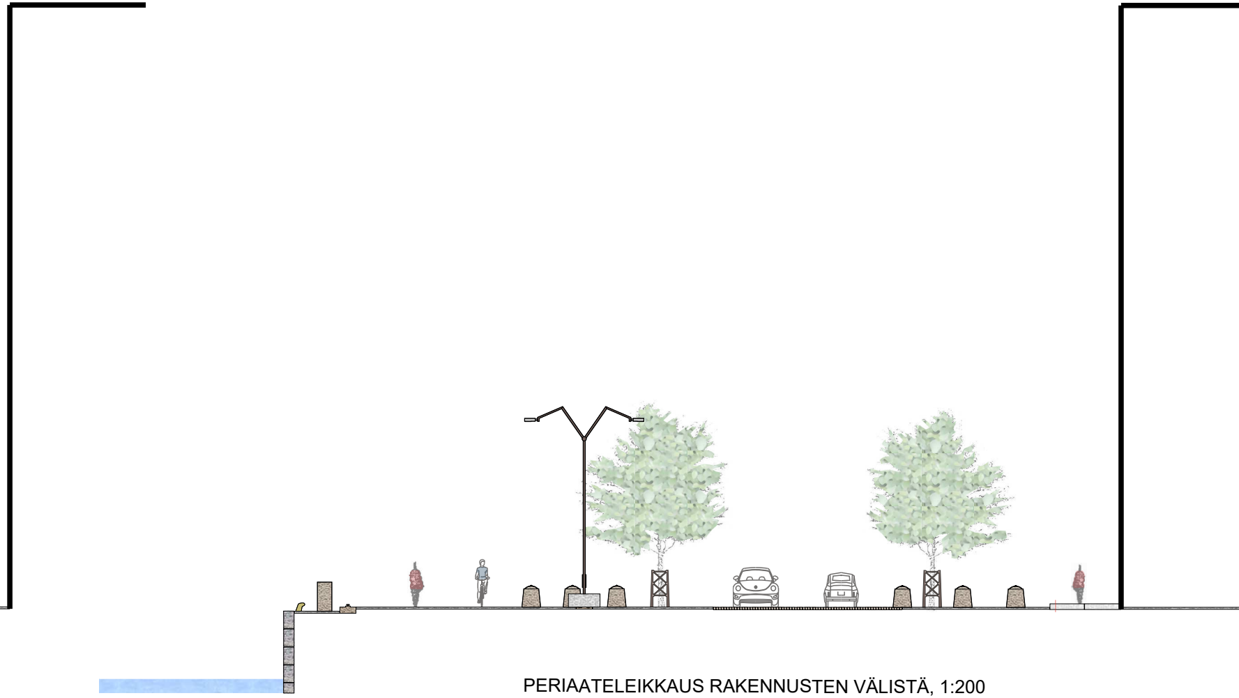
PERIAATELEIKKAUS RAKENNUSTEN VÄLISTÄ, 1:200
