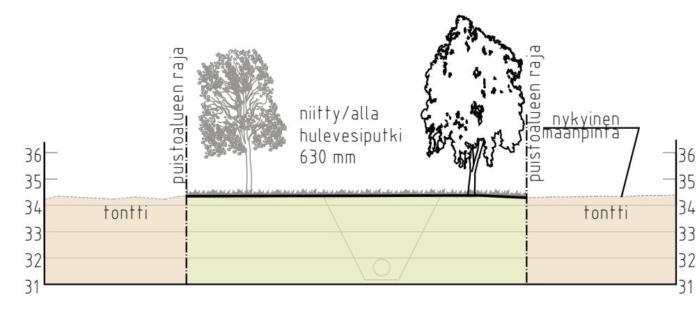
LEIKKAUS A-A
