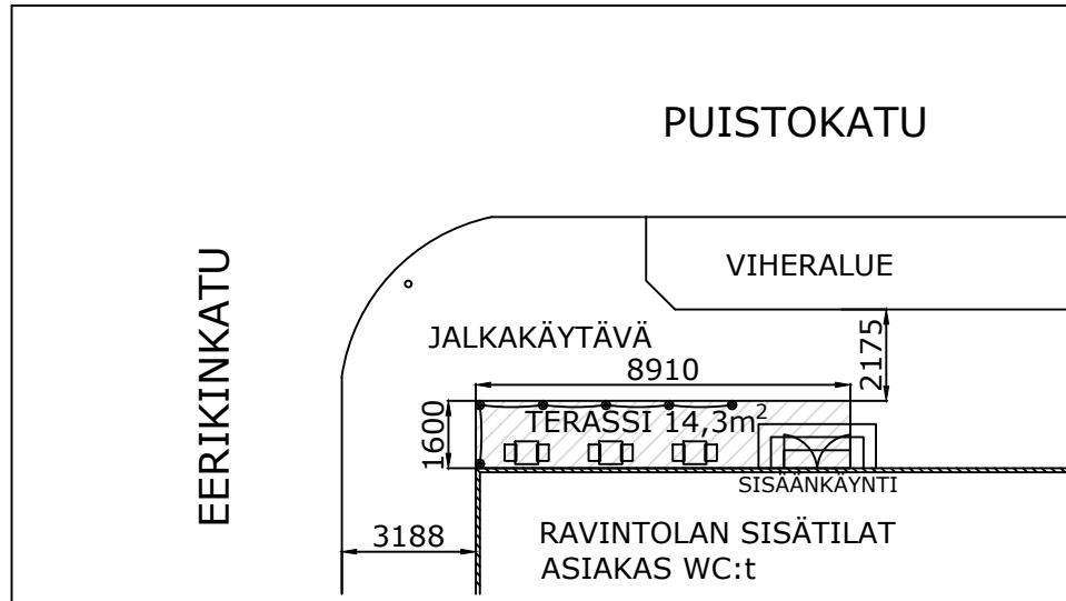
TERASSIALUE 1:200
