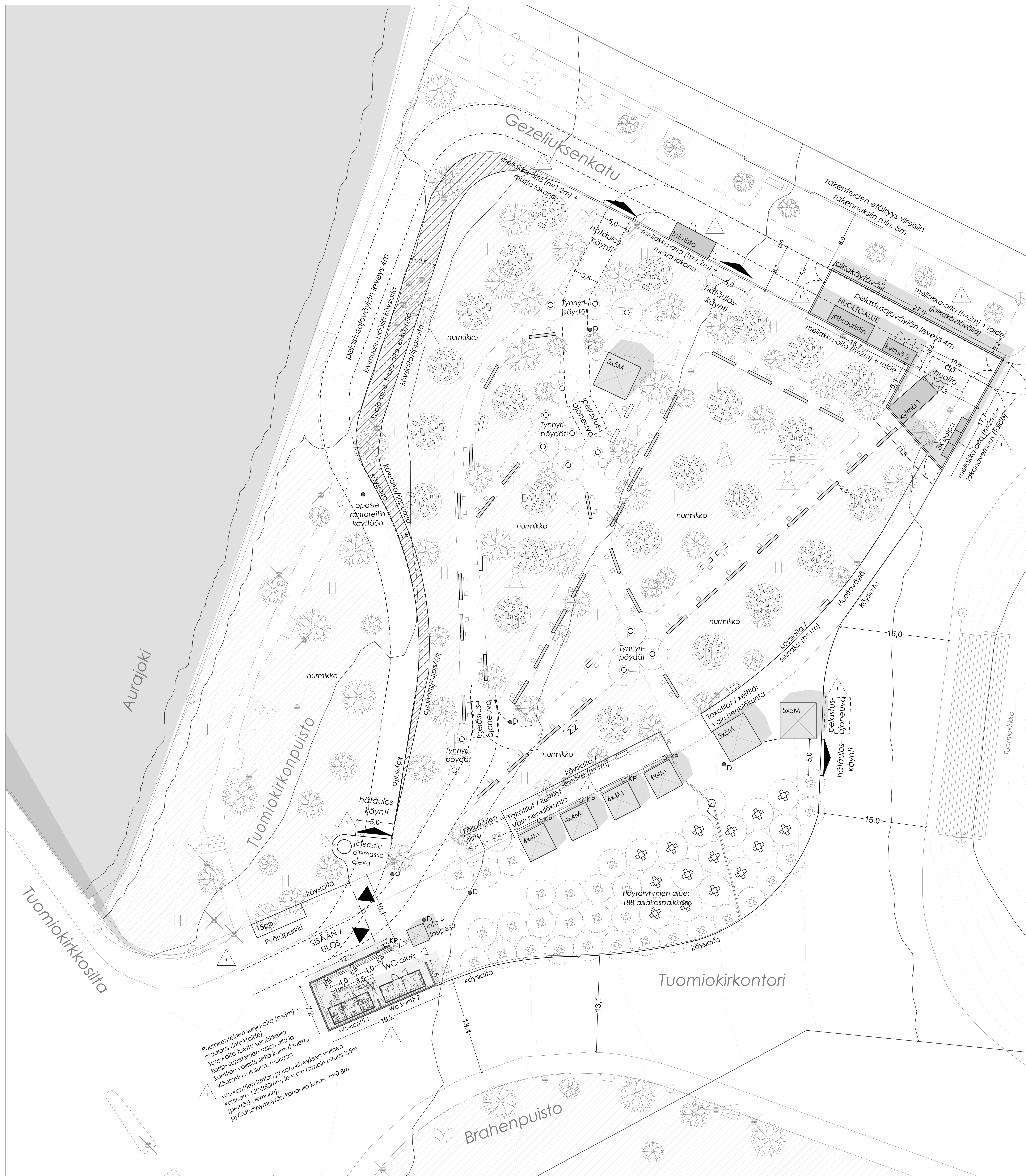
Asemapiirros 1:200
