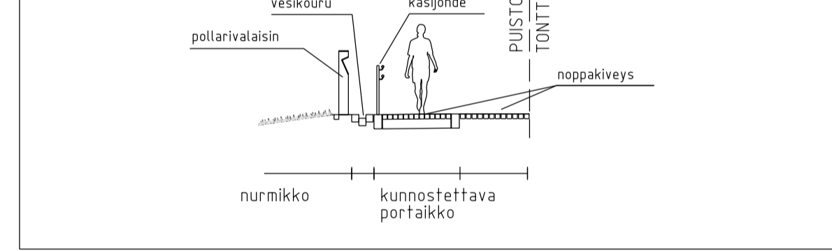
Poikkileikkaus C-C 1:100
