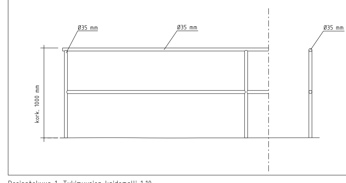
Periaatekuva 1, Tukimuurien kaidemalli 1:10
