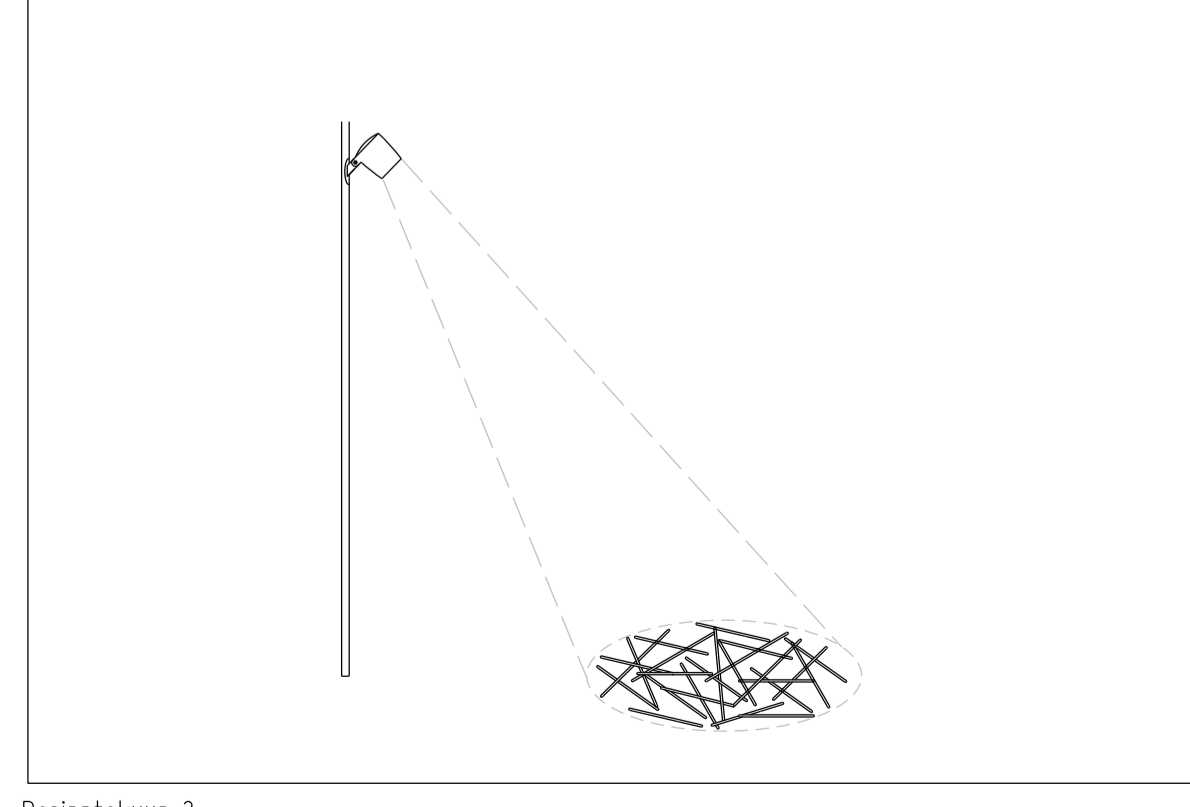
Periaatekuva 2, Kakolanpuiston sisäpuolelaiden valaistusperiaate, jossa profilivalonheittimellä luodaan staattinen kuvio kulkupintaan, ei mittakaavassa.
