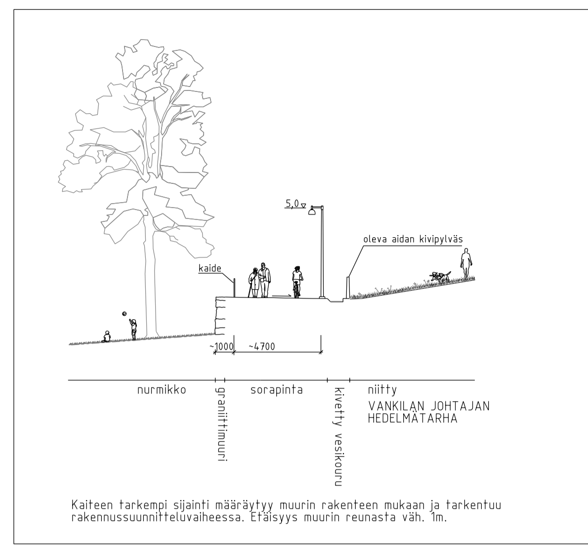
Poikkileikkaus A-A 1:200
