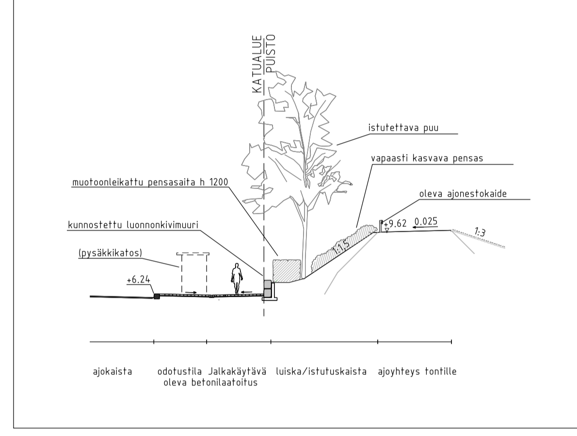
Poikkileikkaus B-B 1:200
