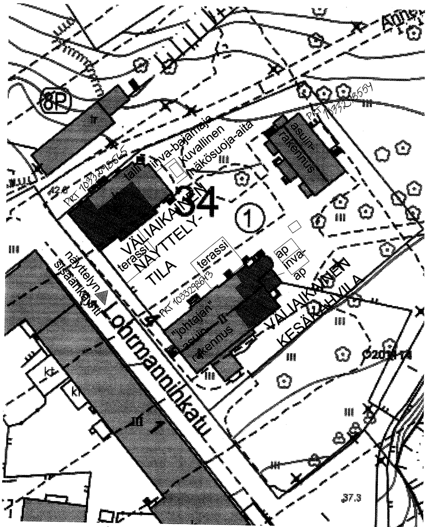
8-34-1 VÄLIAIKAINEN KESÄKAHVILA JA NÄYTTELYTILA ASEMAPUURUUS 1:500
