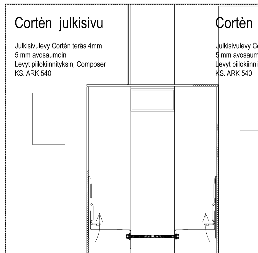
TURVA-AITA 1 DET 01
