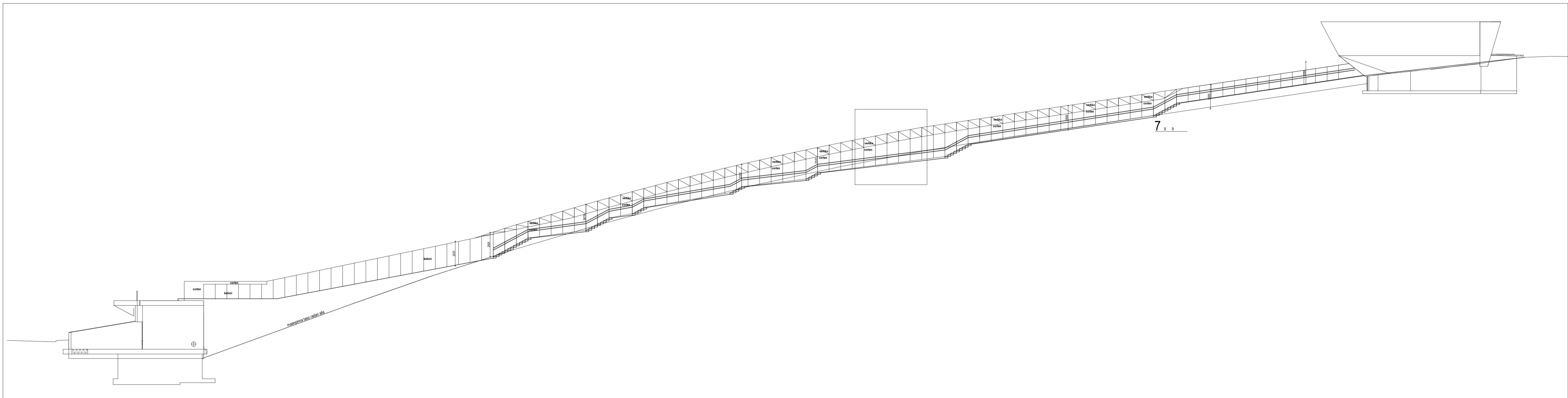
TURVA-AITA 2 Cortén aita integroitu vanhaan portaaseen
