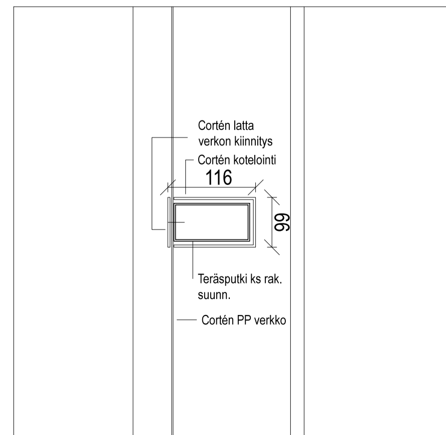
TURVA-AITA 2
