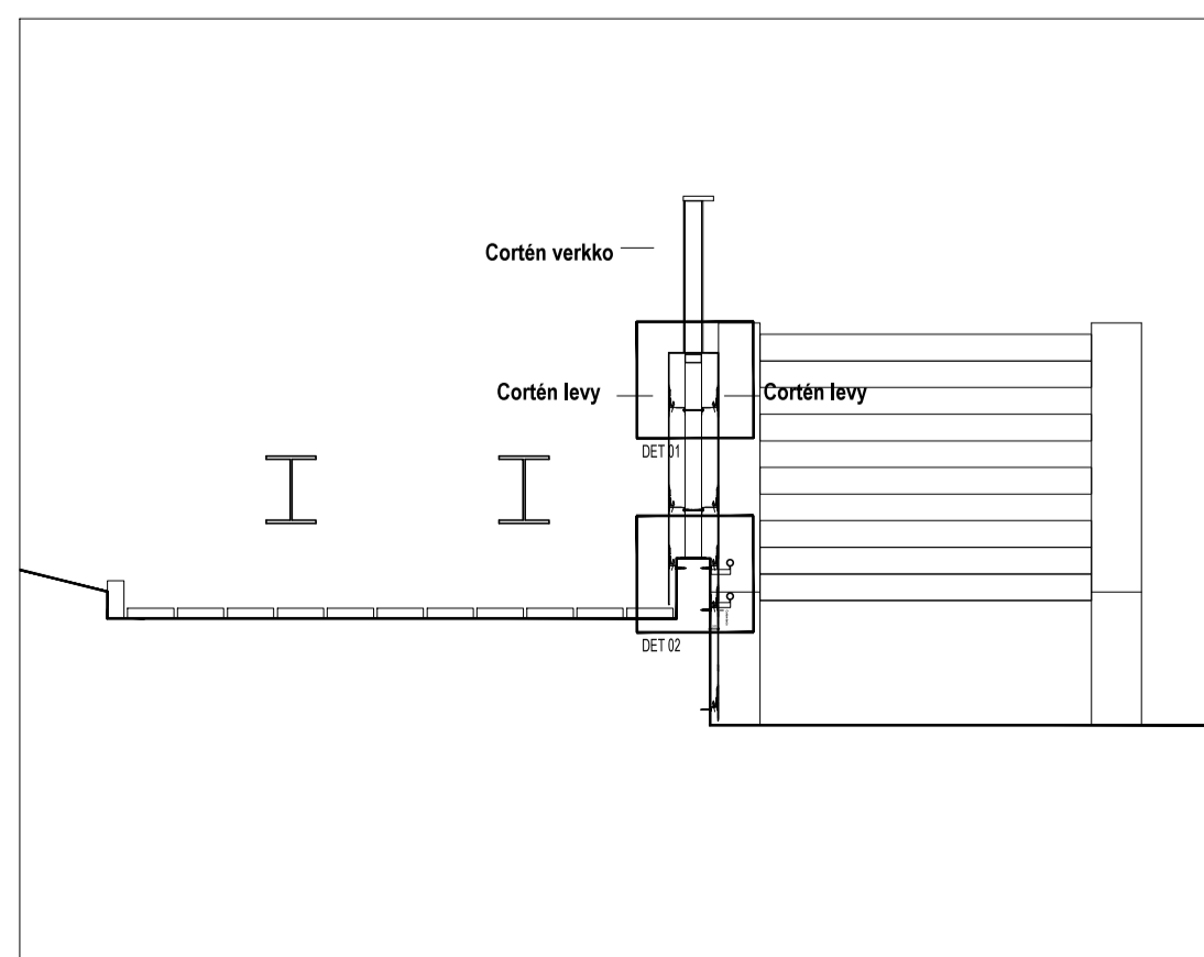
TURVA-AITA 2
