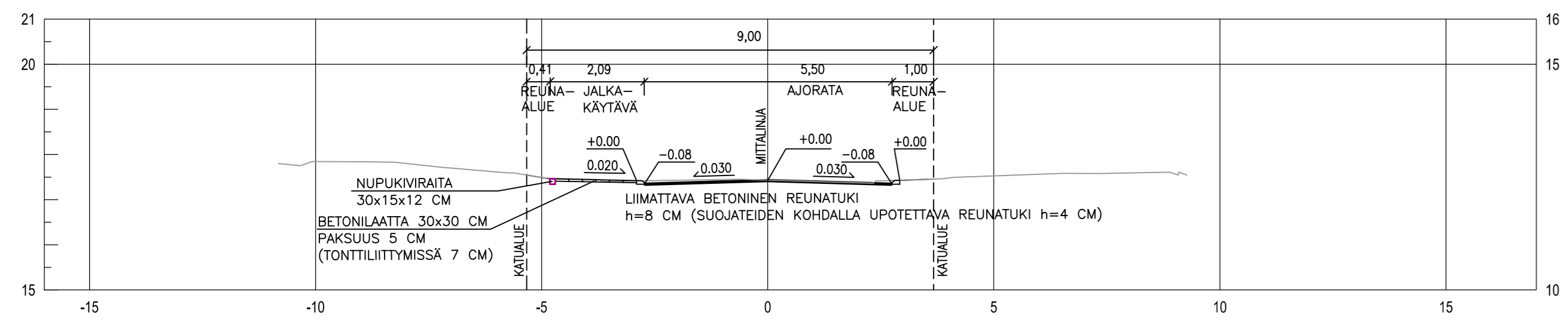
Tyypipoikkileikkaus 1:100
