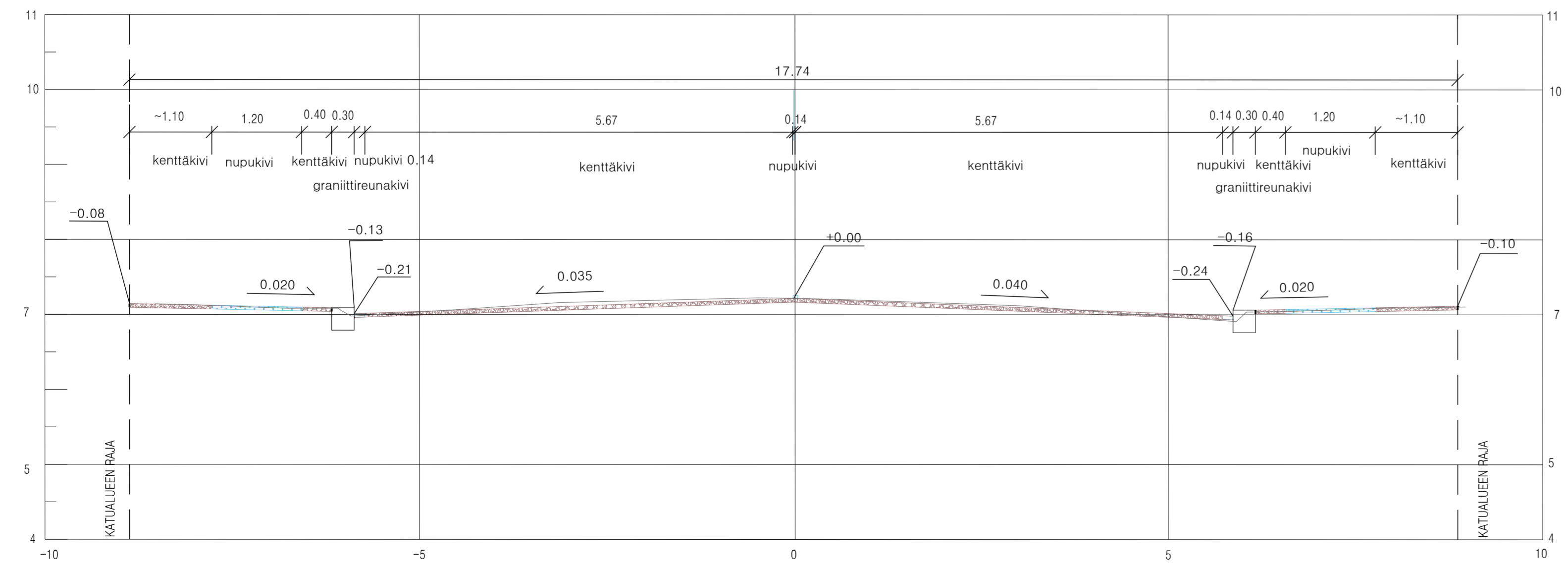
Poikkileikkaus 1:50 PL 60.00
