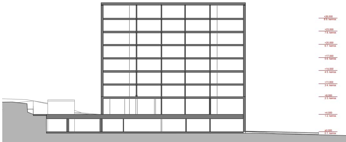
Kuva 44. AK-2, Periaateleikkaus LE 1 Kannuskadulta itään, Arkkitehtitoimisto Matti Takala Oy
