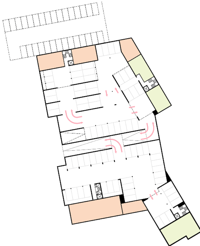
Kuva 57. Periaatekaavio AK-1 -korttelialueen pysäköintijärjestelyistä pihakannen alla. Autopaikkoja on yhteensä 105 kpl (30 kpl maantasossa, 29 kpl rakennusrungoissa ja 46 kpl kahdessa eri tasossa pihakansien alla). Kaaviossa on viitteellisesti esitetty vihreällä kellarikerrokseen sijoittuva rakennusoikeus ja oranssilla rakennusoikeuteen laskemattomat tilat.
