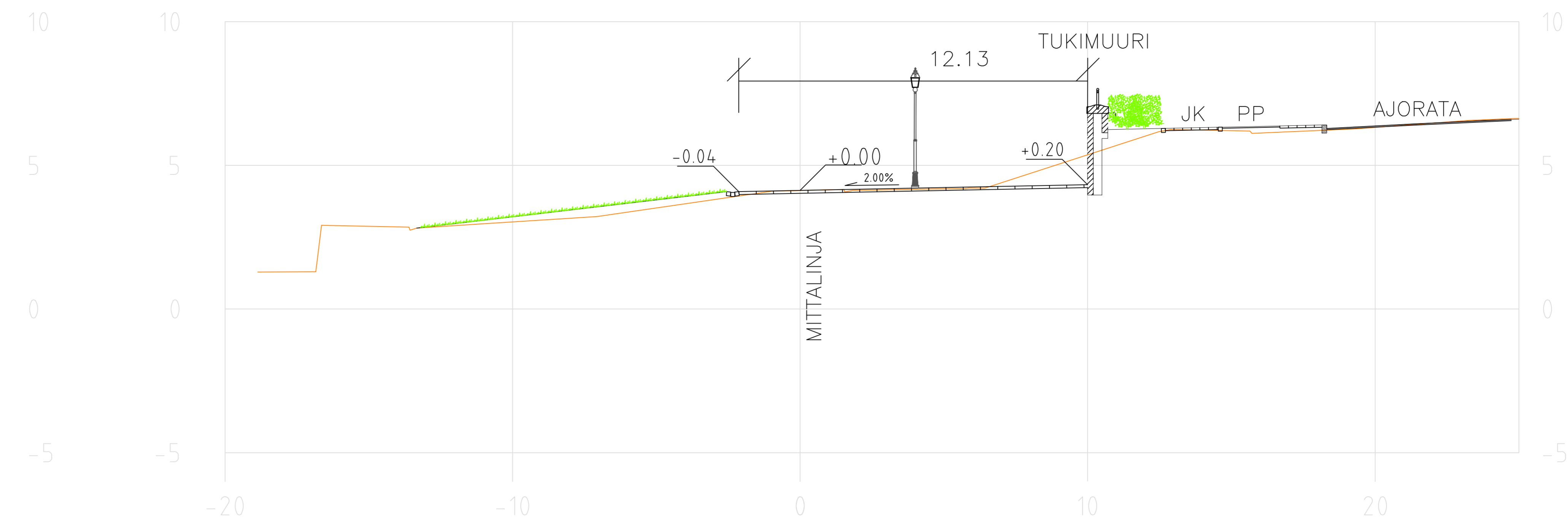
TYYPPIPIIKKILEIKKAUS 1:100 PL 160
