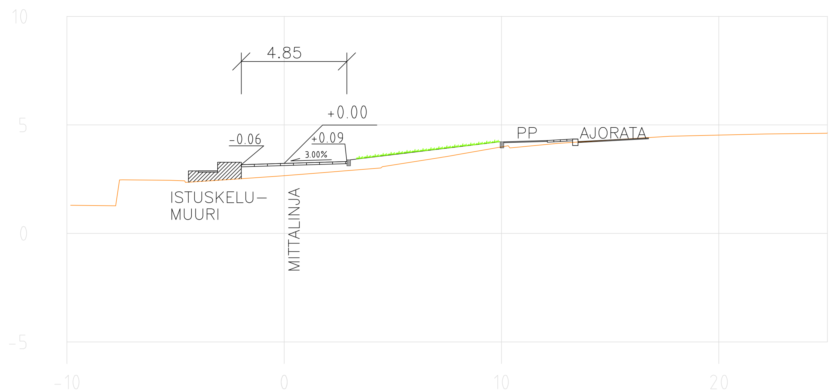
TYYPPIPIIKKILEIKKAUS 1:100 PL 80
