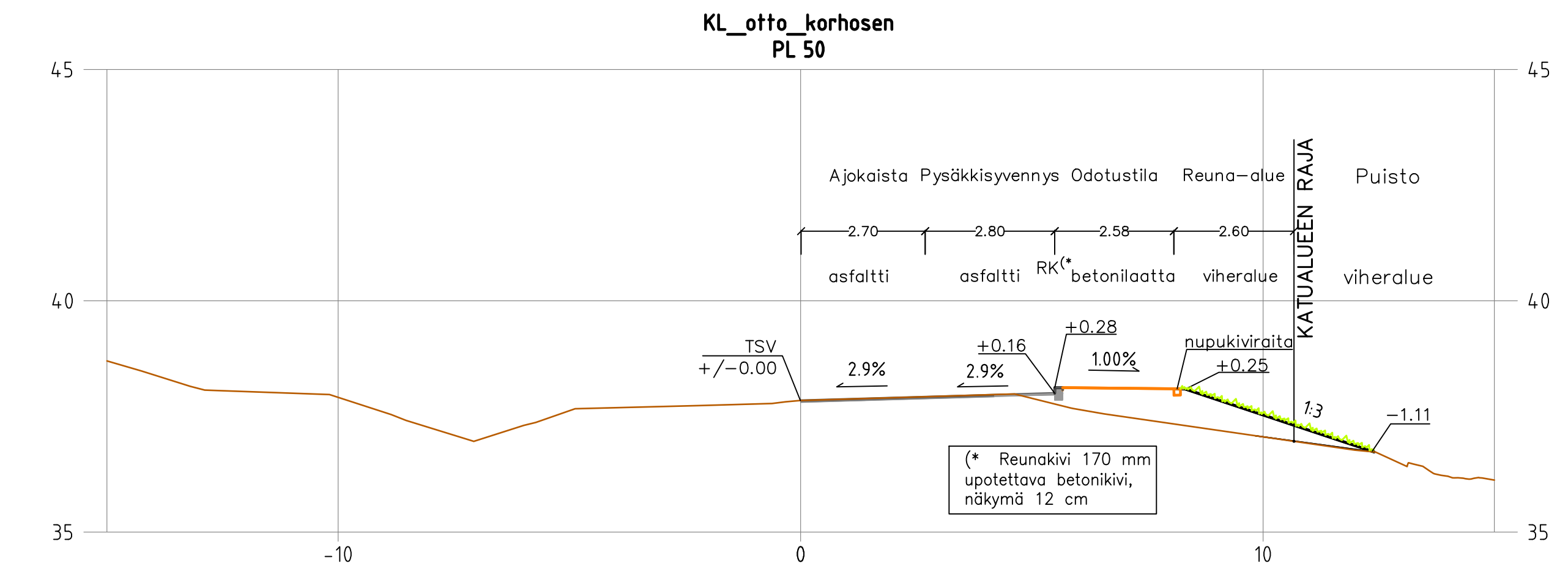
Tyyppiokkeikkaus 1:100 Otto Korhosen katu, pl 50
