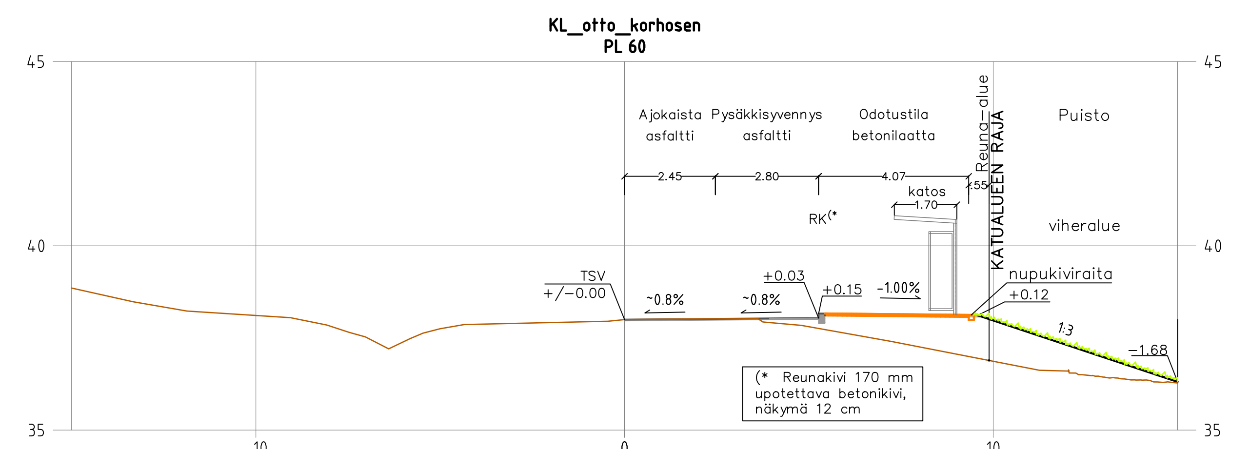
Tyyppiokkeikkaus 1:100 Otto Korhosen katu, pl 60 (linja-autopysäkin katoksen kohta)
