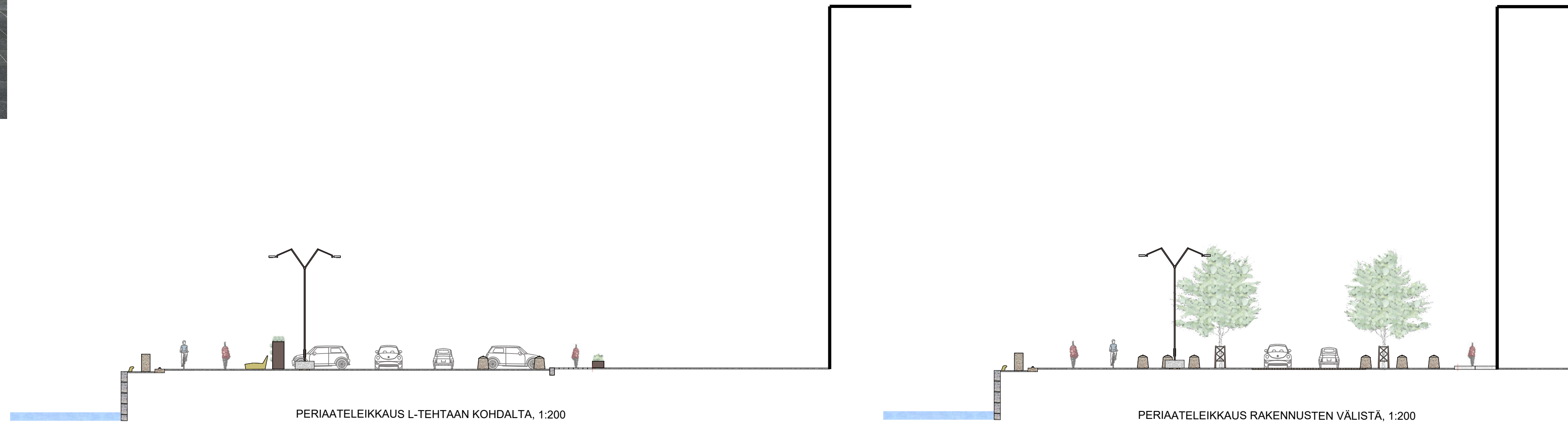
PERIAATELEIKKAUS L-TEHTAAN KOHDALTA, 1:200
