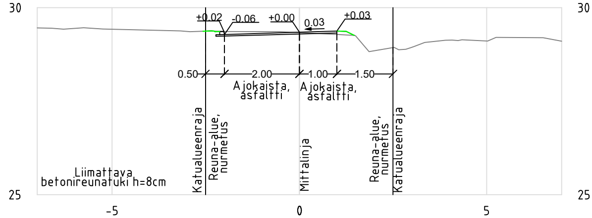
HARJUKATU TYYPPIPOIKKILEIKKAUS 1:100 PL 20.00
