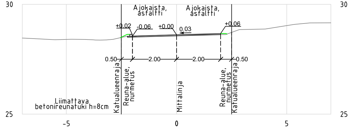
HARJUKATU TYYPPIPOIKKILEIKKAUS 1:100 PL 120.00
