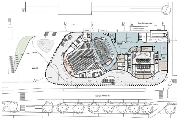
Kuva 24. Konserttitalon 3. kerros, luonnos, PES-Arkkitehdit Oy
