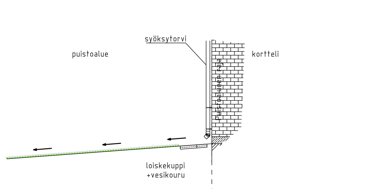
KORTTELIALUEEN HULEVESIEN LIITOSTYYPPI NRÖ 3.
