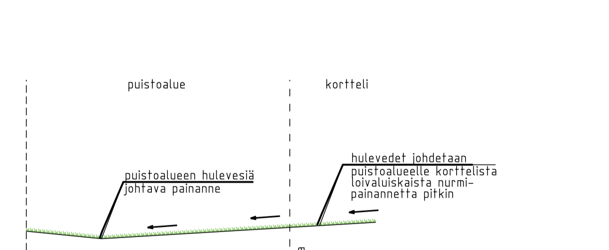
KORTTELIALUEEN HULEVESIEN LIITOSTYYPPI NRÖ 1.
