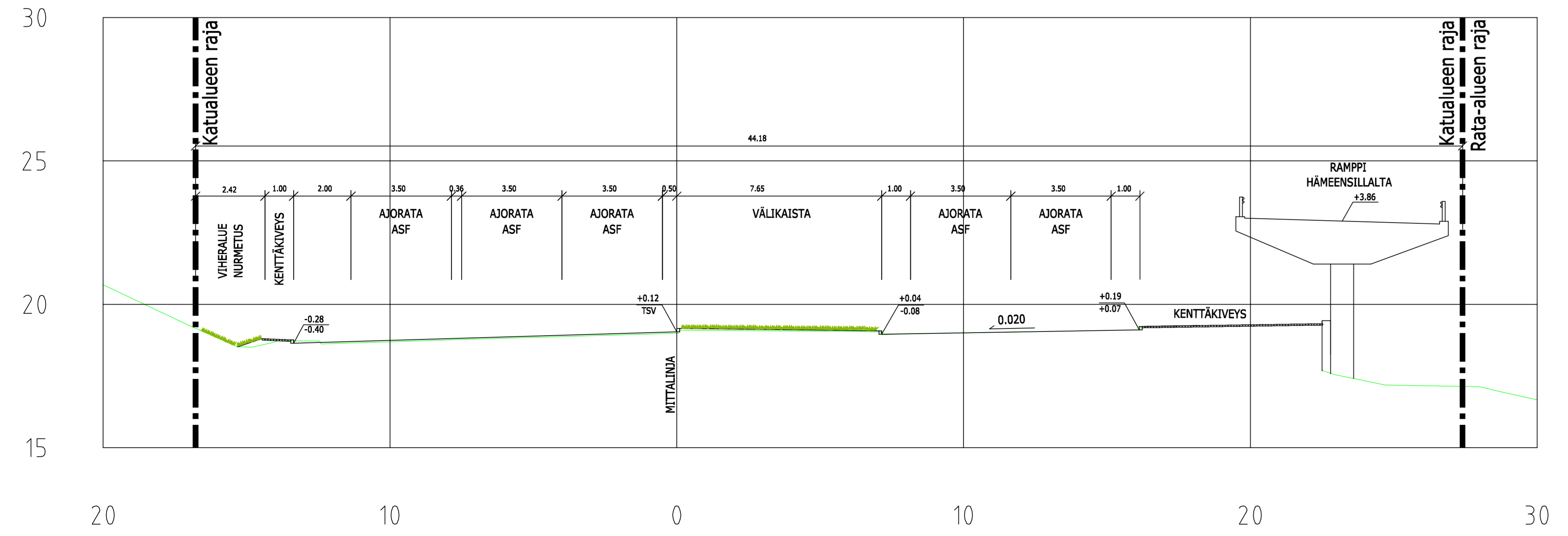
TYYPPIPOIKKILEIKKAUS PAALU 2900 1:100
