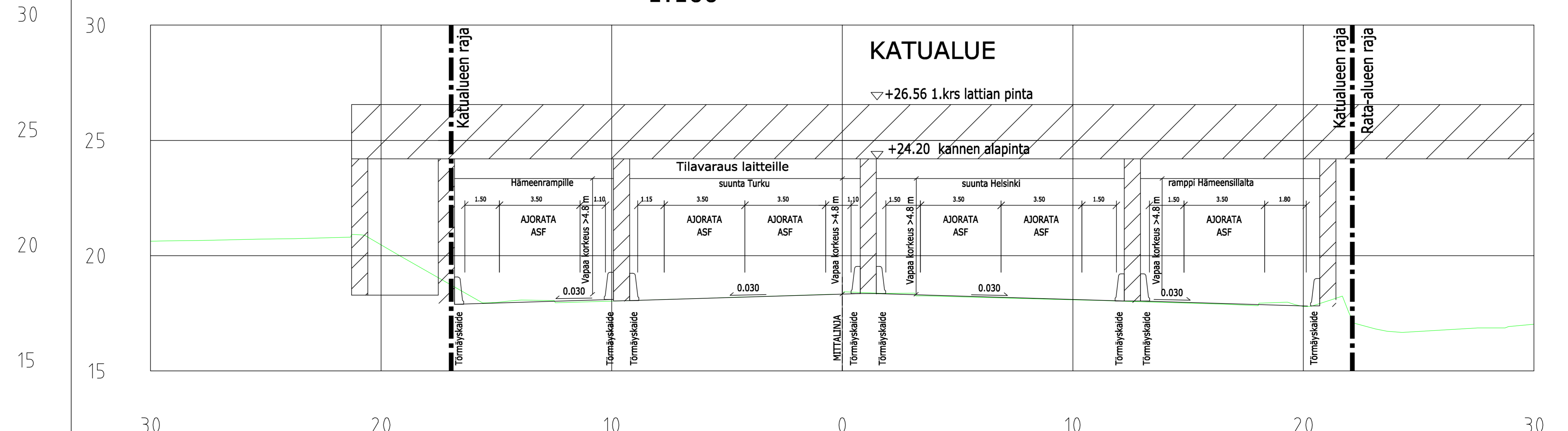
TYYPPIPOIKKILEIKKAUS PAALU 3060 1:100
