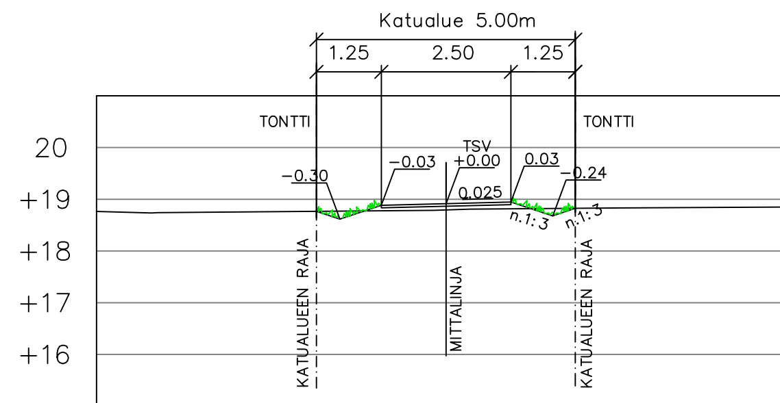
TYYPPIPOIKKILEIKKAUS 1:100 PL 10
