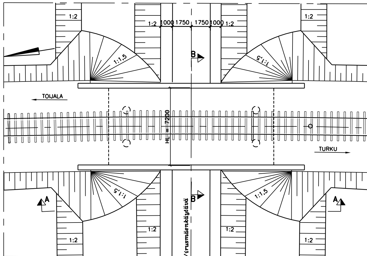
TASOPIIRROS 1:200
