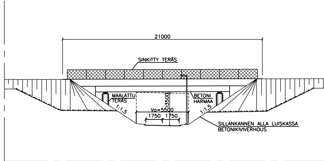
SIVUKUVA A – A, 1:200
