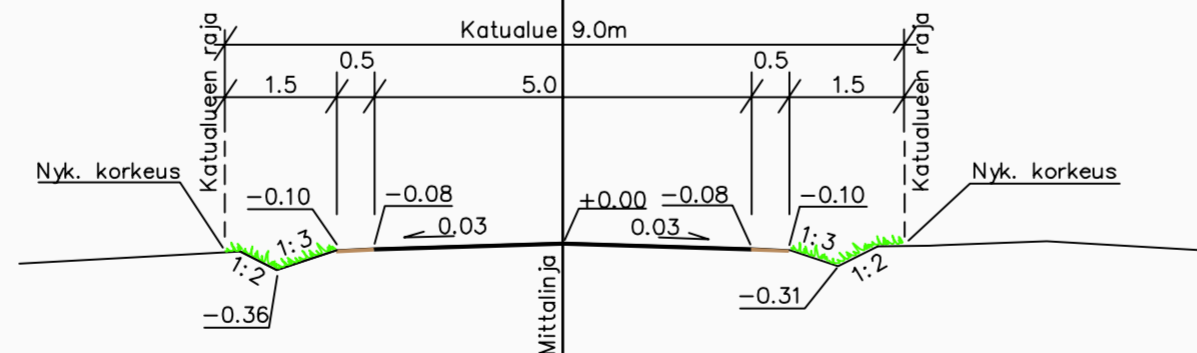
Tyypipoikkileikkaus 1:100 PL 560
