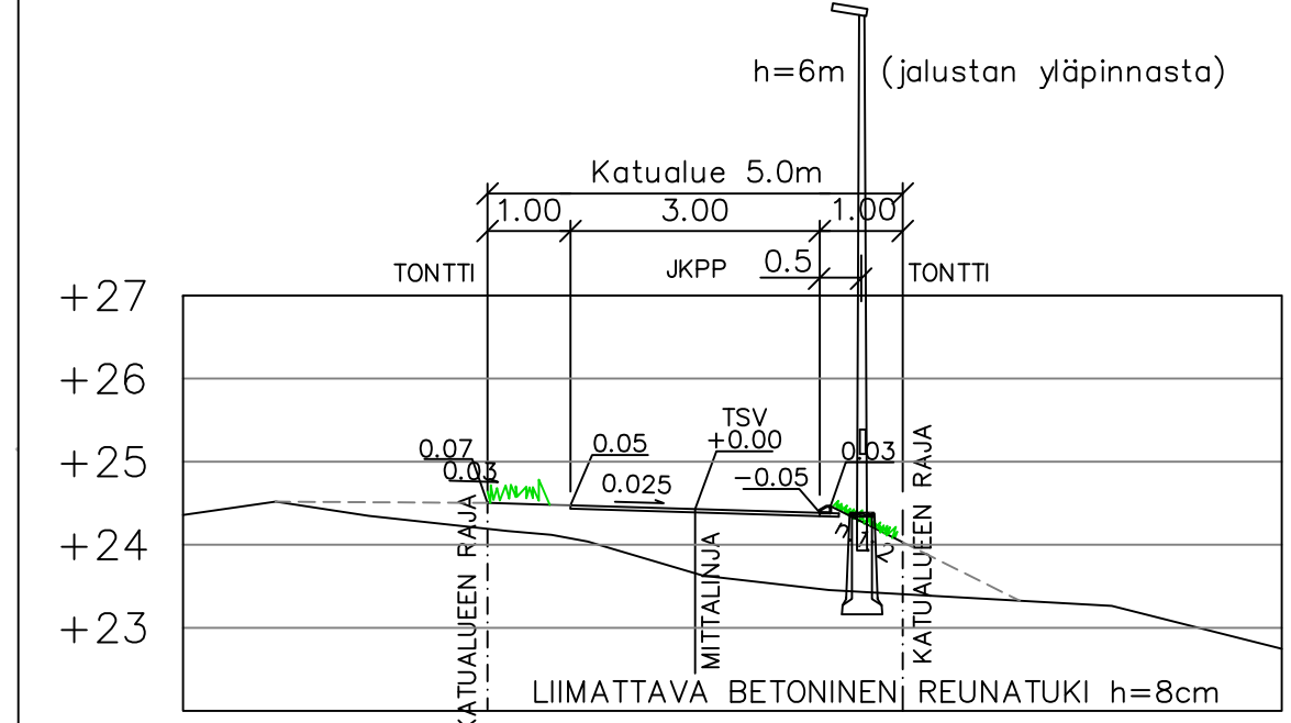
TYYPPIPOIKKILEIKKAUS 1:100 PL 40
