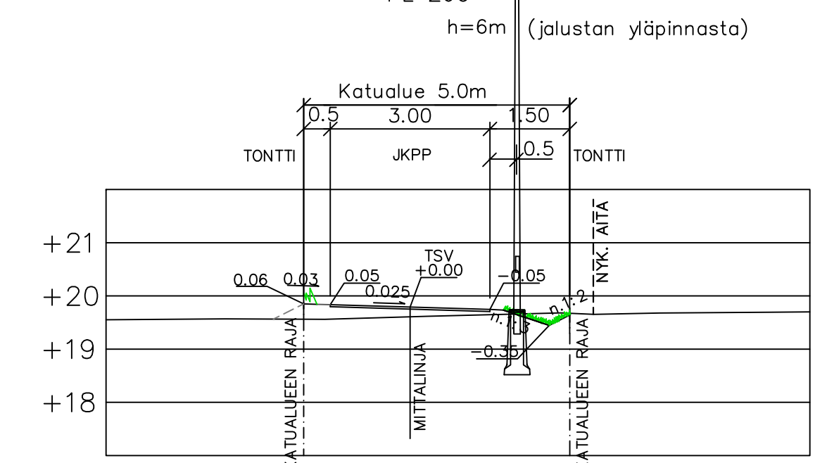
TYYPPIPOIKKILEIKKAUS 1:100 PL 260
