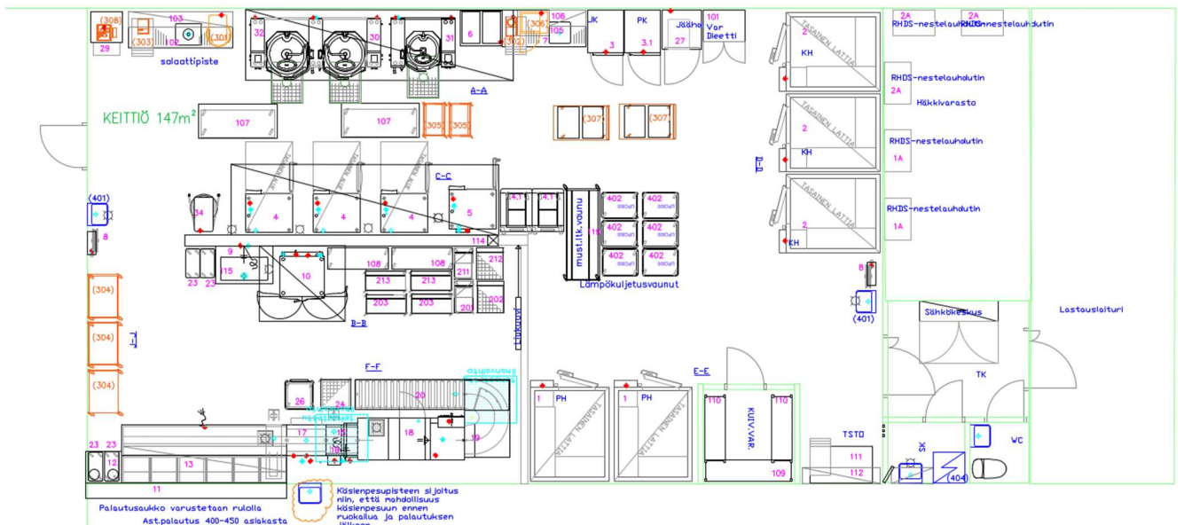
Kuva 6, malli valmistuskeittiökonepohjakuva.
