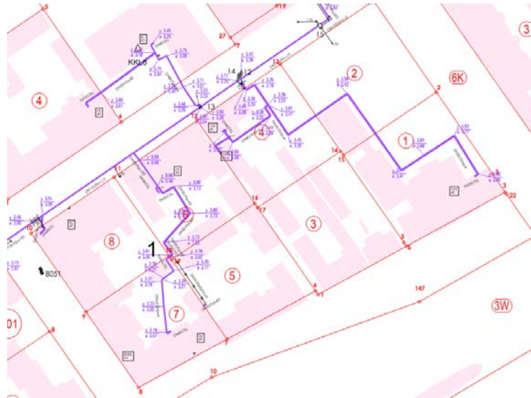
kaukolämpöputket
