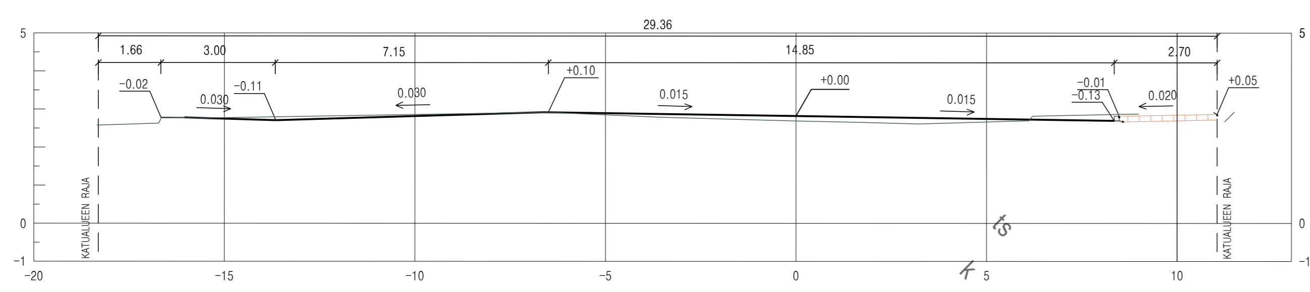
Tyyppipoikkileikkaus 1:100 PL 640.00
