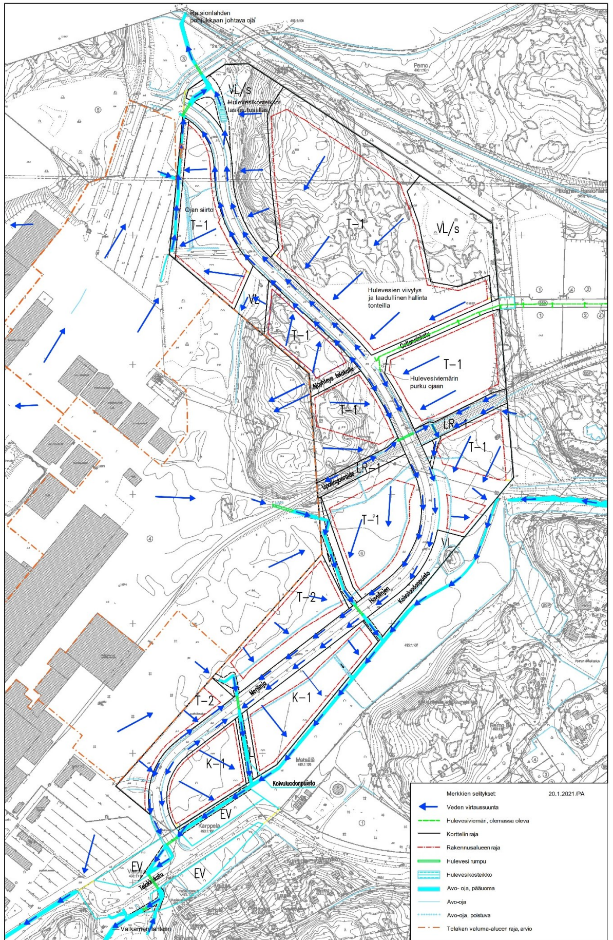
Kuva 18. Periaatekuva hulevesijärjestelyistä
