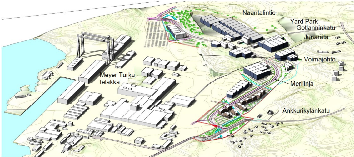
Kuva 17. Kaavuluonnoksen havainnekuva
