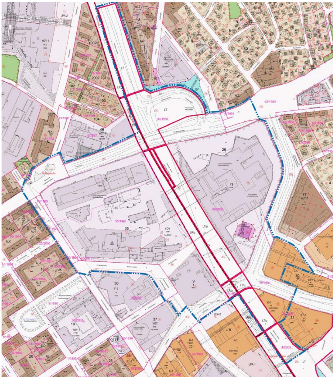
Ajantasa-asemakaava 12.2.2015
